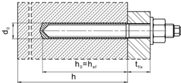
Abbildung A1: Gewindestange, HAS..., HAS-U..., HAS-..., HIT-V..., AM...8.8
